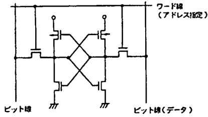
スイッチ設定用PROM50の内部回路図 第4図(B)
